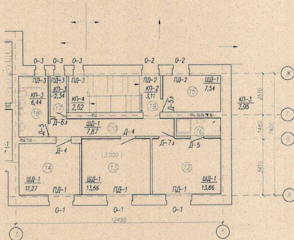
План 2 этажа д.№18
