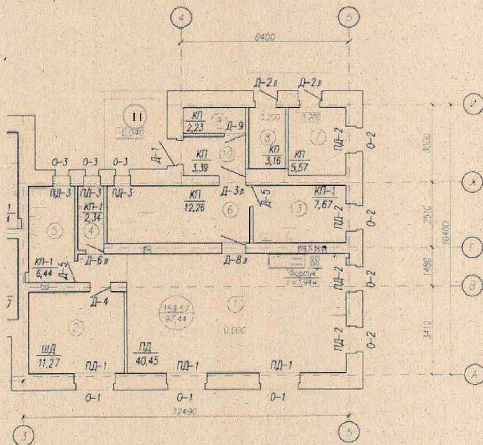
План 1 этажа д.№18
